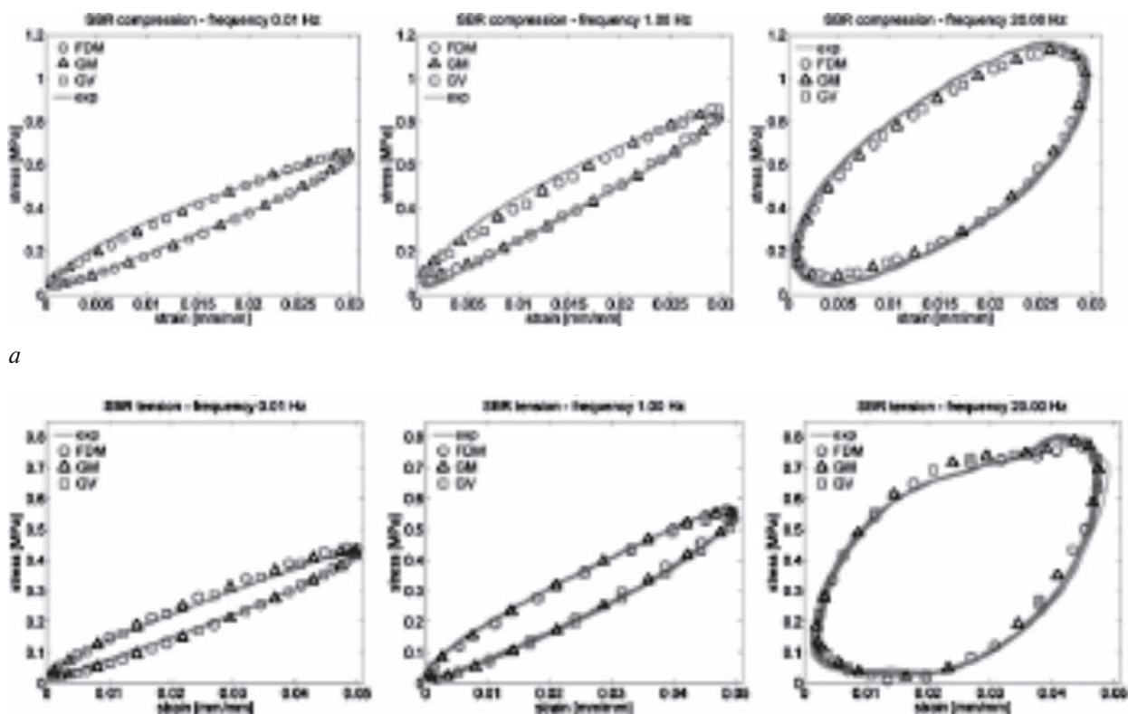
Рисунок 1 — Адекватность использования моделей, построенных на основе математического аппарата дробного интегро-дифференцирования: a — кривая гистерезиса образцов I вида при 0,01 Гц, 1,00 Гц, 20,00 Гц; б — кривая гистерезиса образцов II вида при 0,01 Гц, 1,00 Гц, 20,00 Гц
