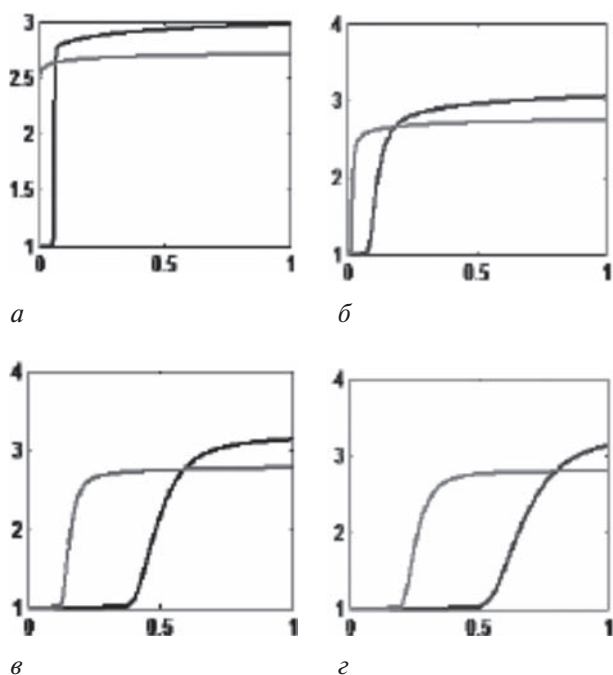
Рисунок 3 — Поведение изотропной функции роста g(t) при значениях (адаптирован из [30]):
