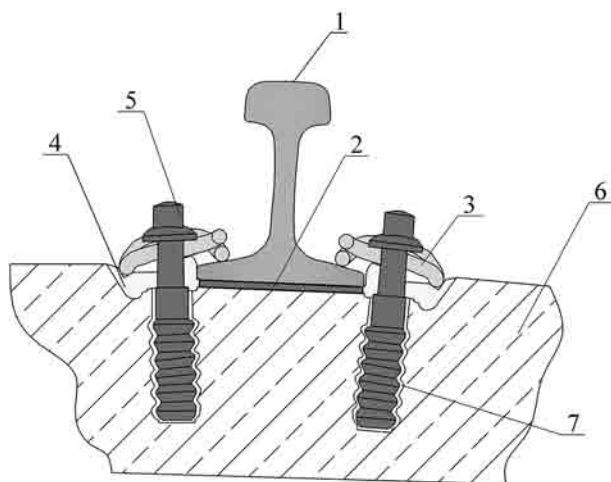
Рисунок 6 — Общий вид рельсового скрепления фирмы Vossloh:
